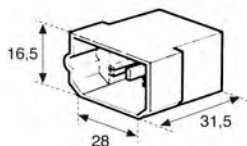
• 4 way male.
